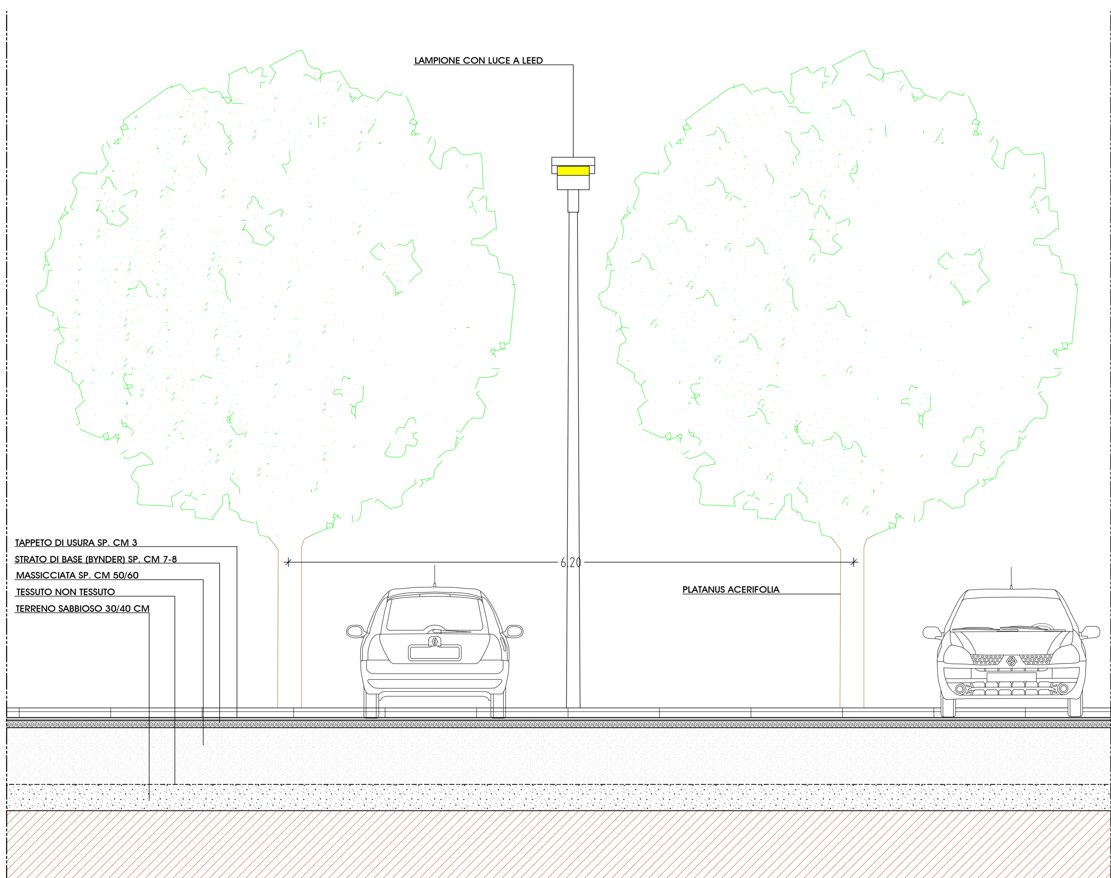
PARTICOLARE ② VISTA IN PROSPETTO AREA VERDE TRA I PARCHEGGI Scala 1:25
