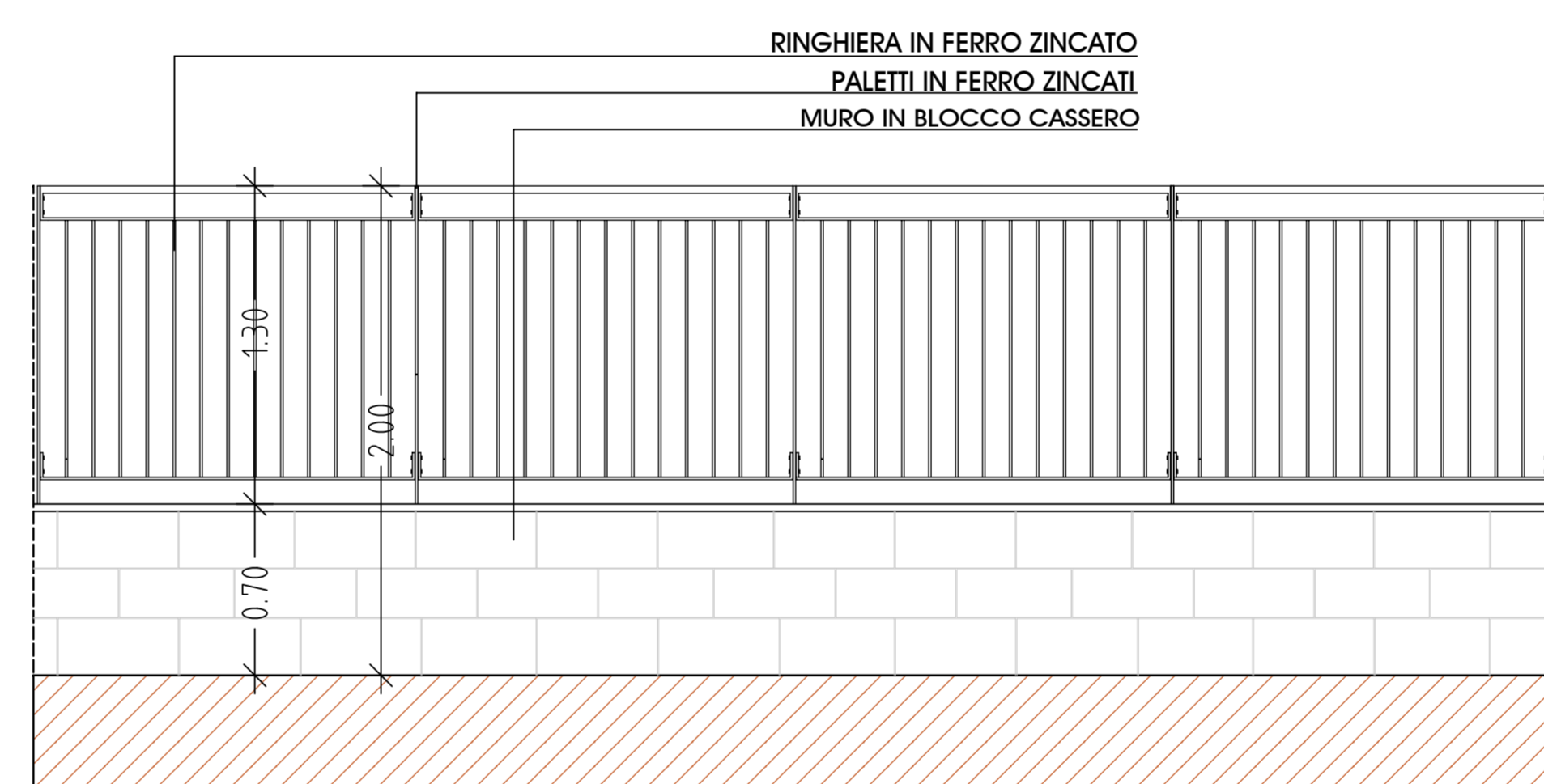
PARTICOLARE ③ MURETTO CON RINGHIERA IN FERRO ZINCATO Scala 1:25
