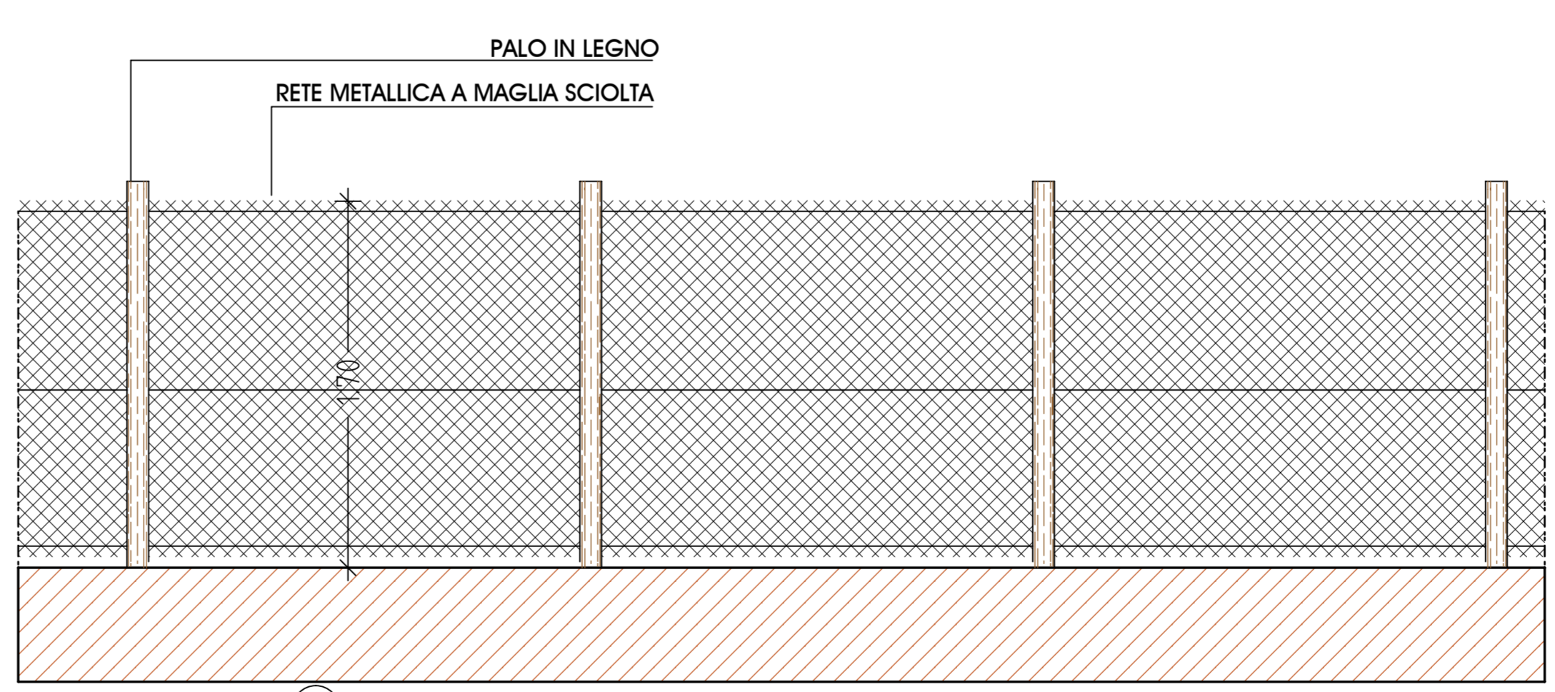
PARTICOLARE ④ RECINZIONE CON PALI IN LEGNO E RETE METALLICA Scala 1:25
